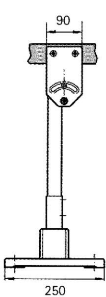
Floor stand FZK121
