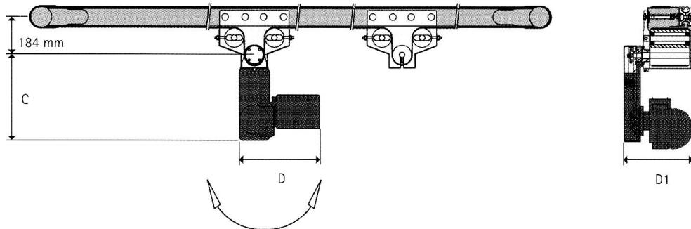
FK120 keskimoottorilla ja kiristyslaitteella (5000mm:stä eteenpäin)
